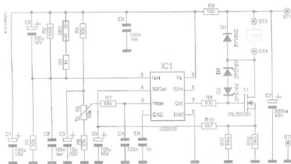
Abb. 70: Schaltbild der PWM 2. Generation
