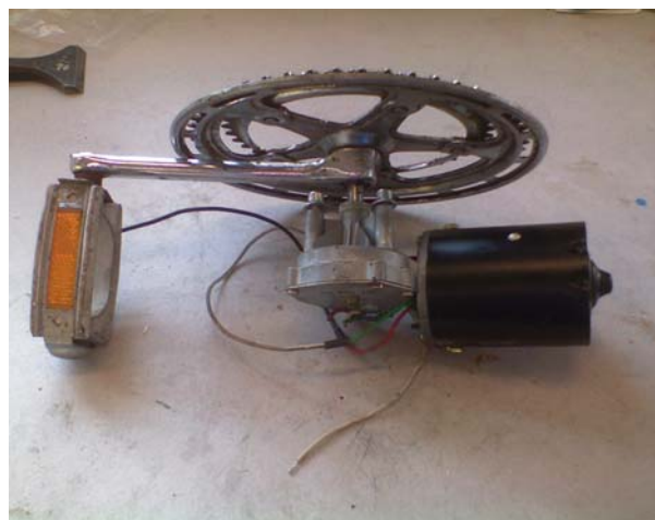
Abb. 41: Montagesystem
