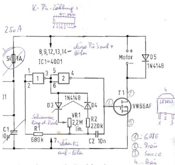
Abb. 64: Schaltbild der PWM 1. Generation
