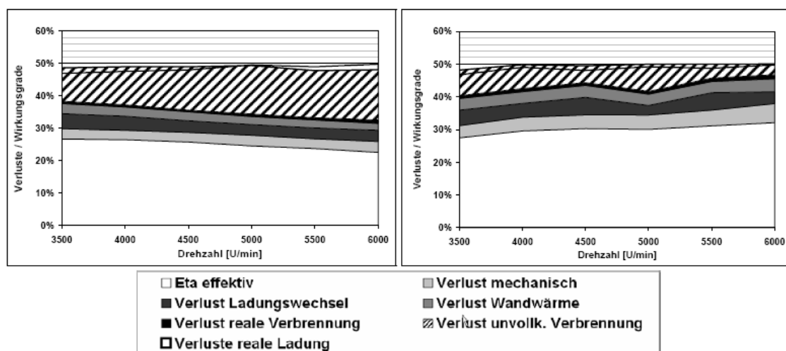
Abb. 2: Wirkungsgrade und Wirkungsgradverluste von 2-Takt-Motoren, bei früher Einspritzung (links) und später Einspritzung (rechts) [A2]
