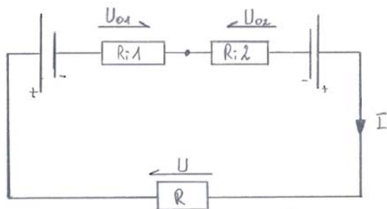
Abb. 77: Schaltbild Gegenreihenschaltung
